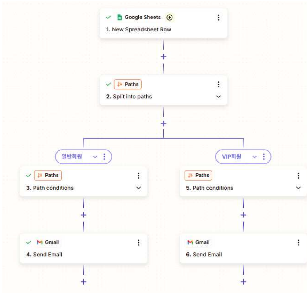
그림 4. Zapier 회원 안내 이메일 자동화 전체 화면
