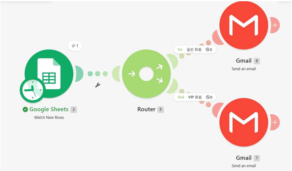
그림 1. Make 회원 안내 이메일 자동화 전체 화면
